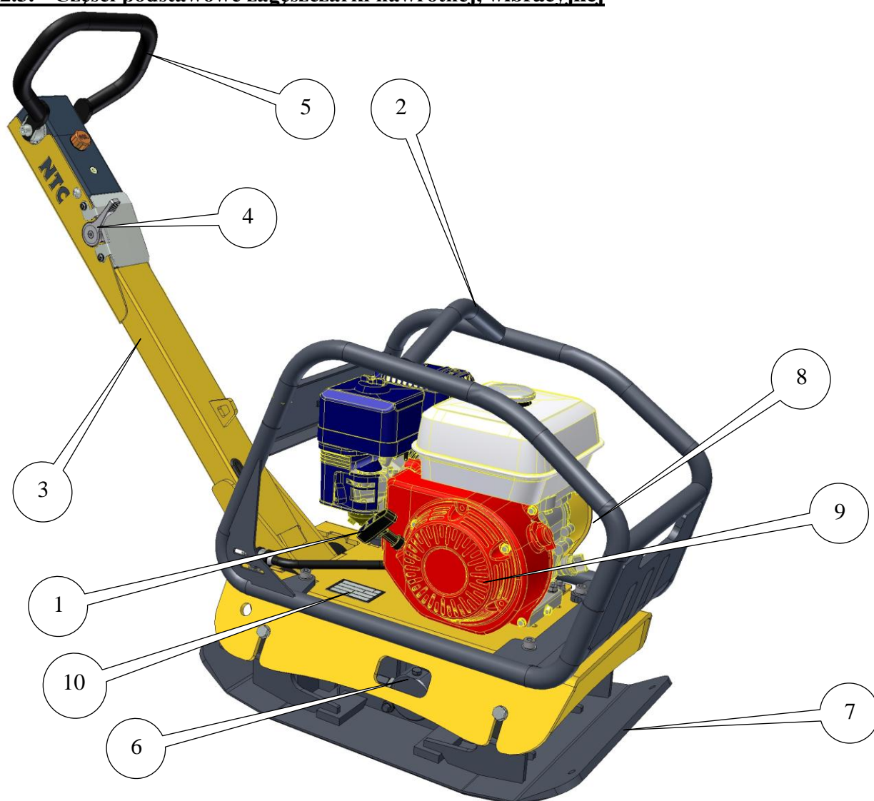
Części podstawowe zagęszczarki nawrotnej, wibracyjnej:
